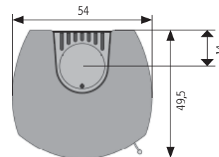
bovenaanzicht
