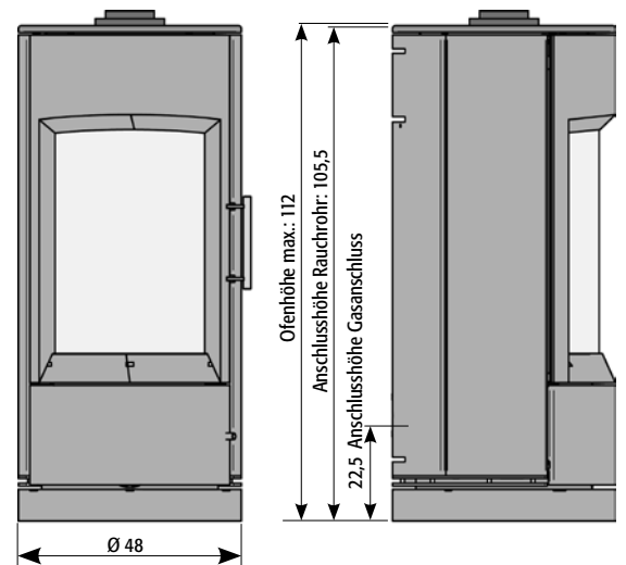
Vorderansicht
